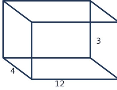
Ayrıtları 3, 4 ve 12 olan dikdörtgenler prizması
