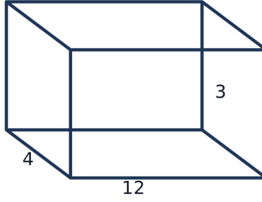
Ayritları 3, 4 ve 12 olan dikdörtgenler prizması
